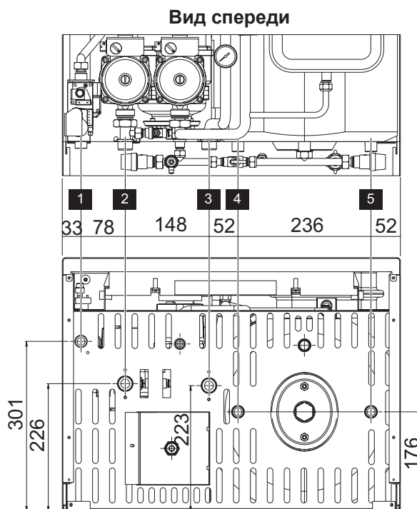
Вид снизу
